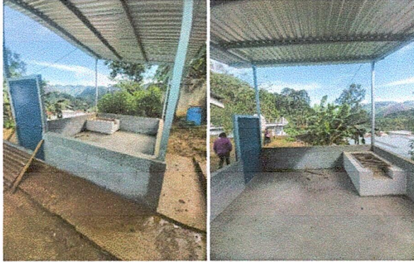
Foto 1: MEJORAMIENTO INSTALACIÓN ESTRUCTURA PORTANTE (TIPO PORTICO) Y CUBIERTA TECHO LÁMINA TROQUELADA CALIBRE 26 (AREA DE COCINA), MEJORAMIENTO DE LOSA DE PATIO
