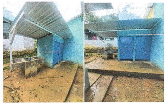
Foto 2: MEJORAMIENTO DE PUERTAS Y CUBIERTA SERVICIOS SANITARIOS
